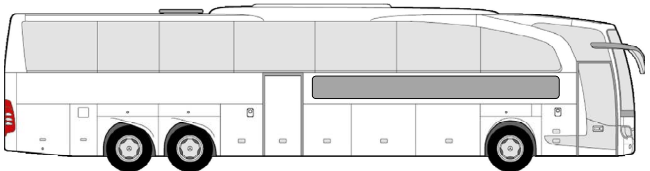
Länge: 13,00 Meter / Breite: 2,55 Meter / Höhe: 3,75 Meter
